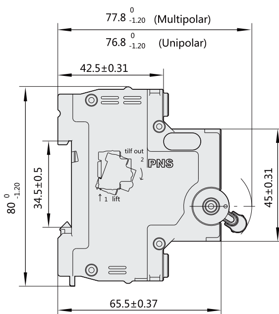
ابعاد کلی کلیدهای مینیاتوری
